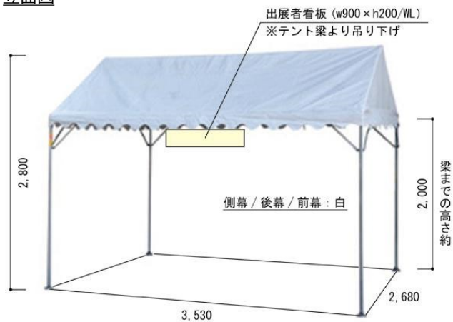
立面図
